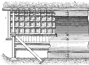
LONGITUDINAL SECTION.
